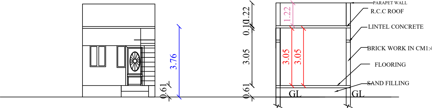
ELEVATION
