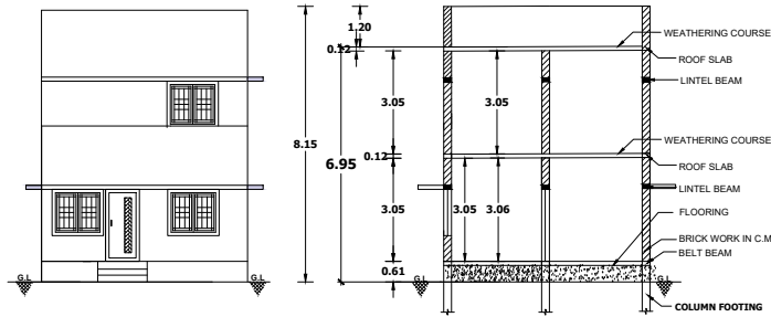
ELEVATION
