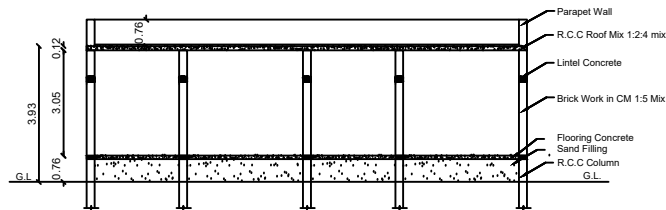
ELEVATION
