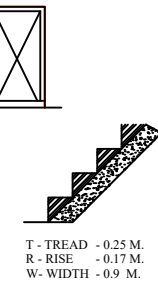
STAIRCASE DETAILS - N.T.S
