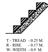
STAIRCASE DETAILS - N.T.S
