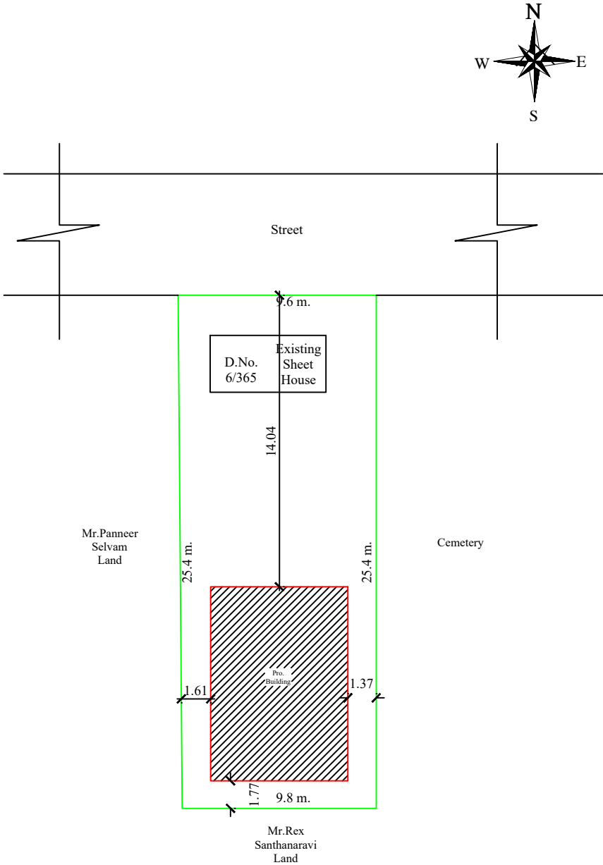
SITE PLAN 1:200
