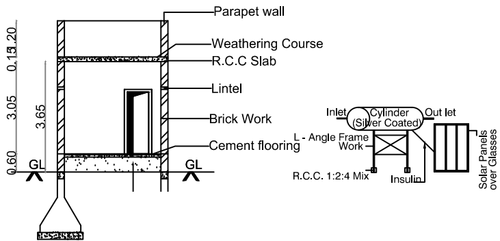
SECTIC (SCALE: 1"=1'-0")
