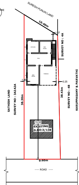
SITE PLAN ( SCALE : - 1:200 )
