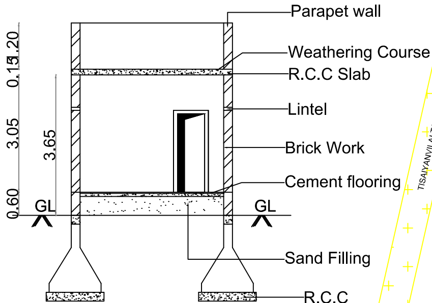
SECTION : "A-A" (SCALE: 1CM : 1M)
