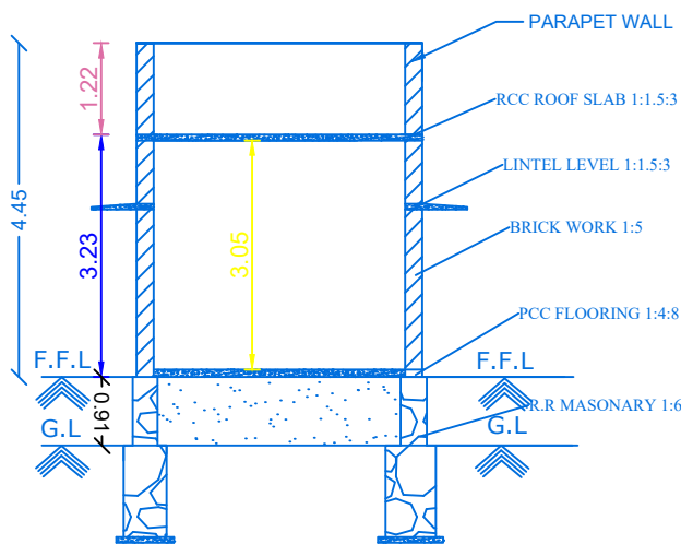
SECTION A-B
