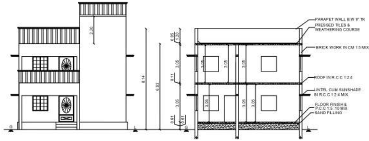
ELEVATION
