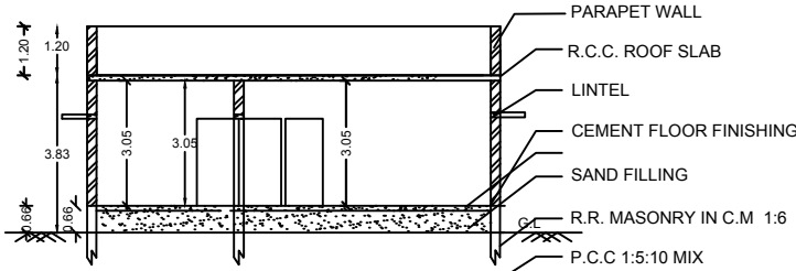
SECTION - AB
