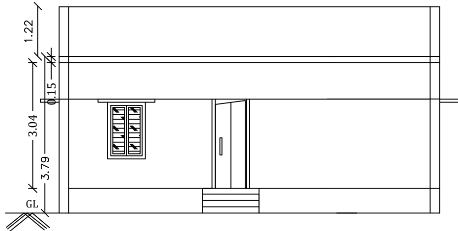
ELEVATION
