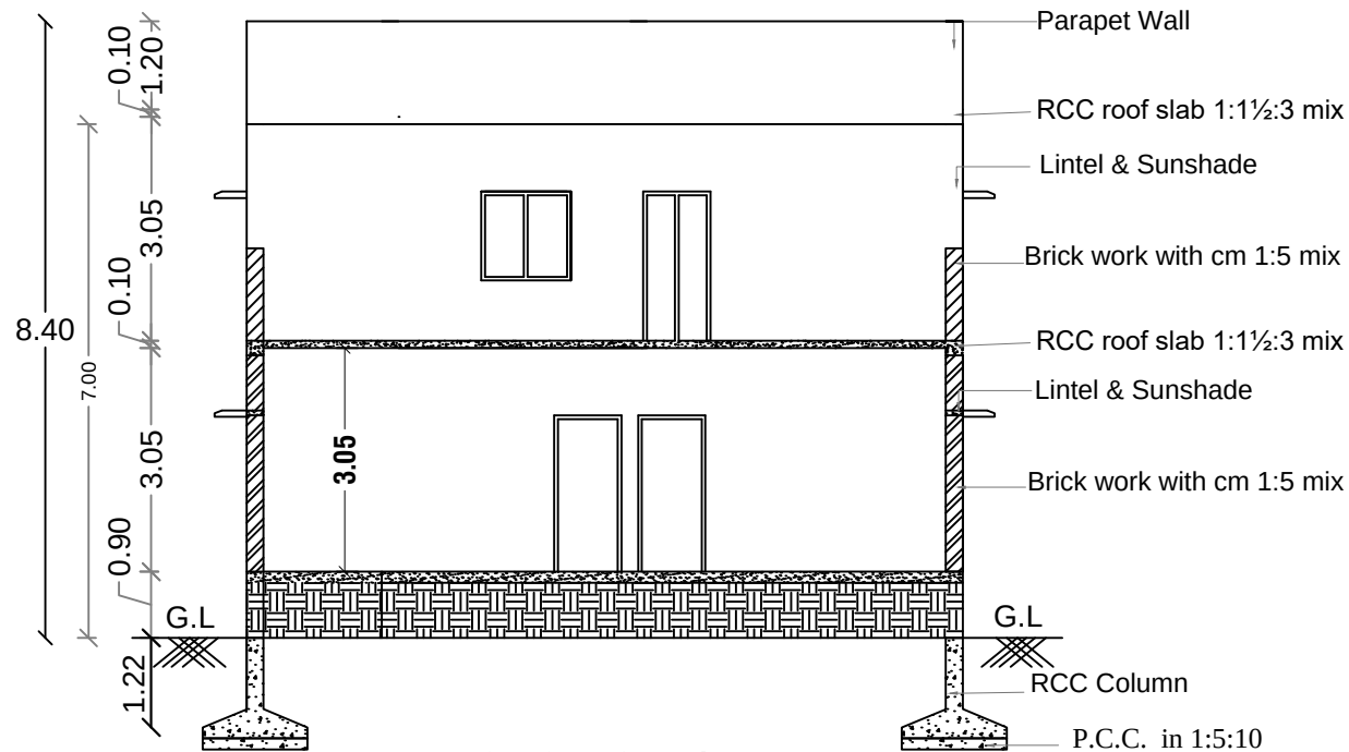
SECTION A-B
