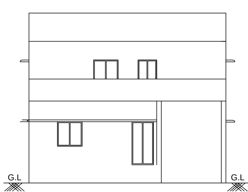
ELEVATION
