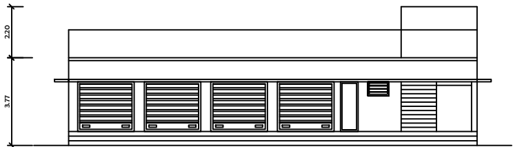
ELEVATION
