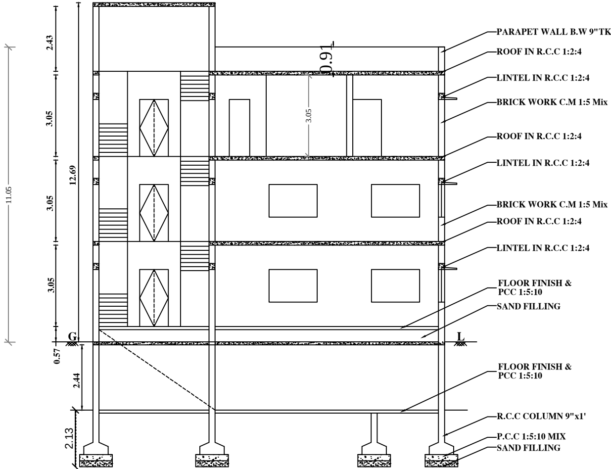
SECTION A-A'
