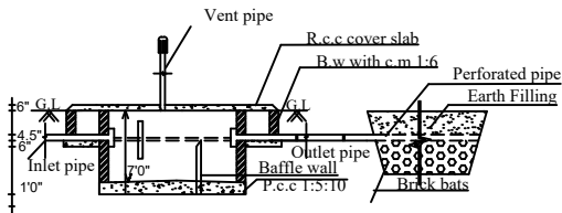
SECTION OF S.P.T & D.T
