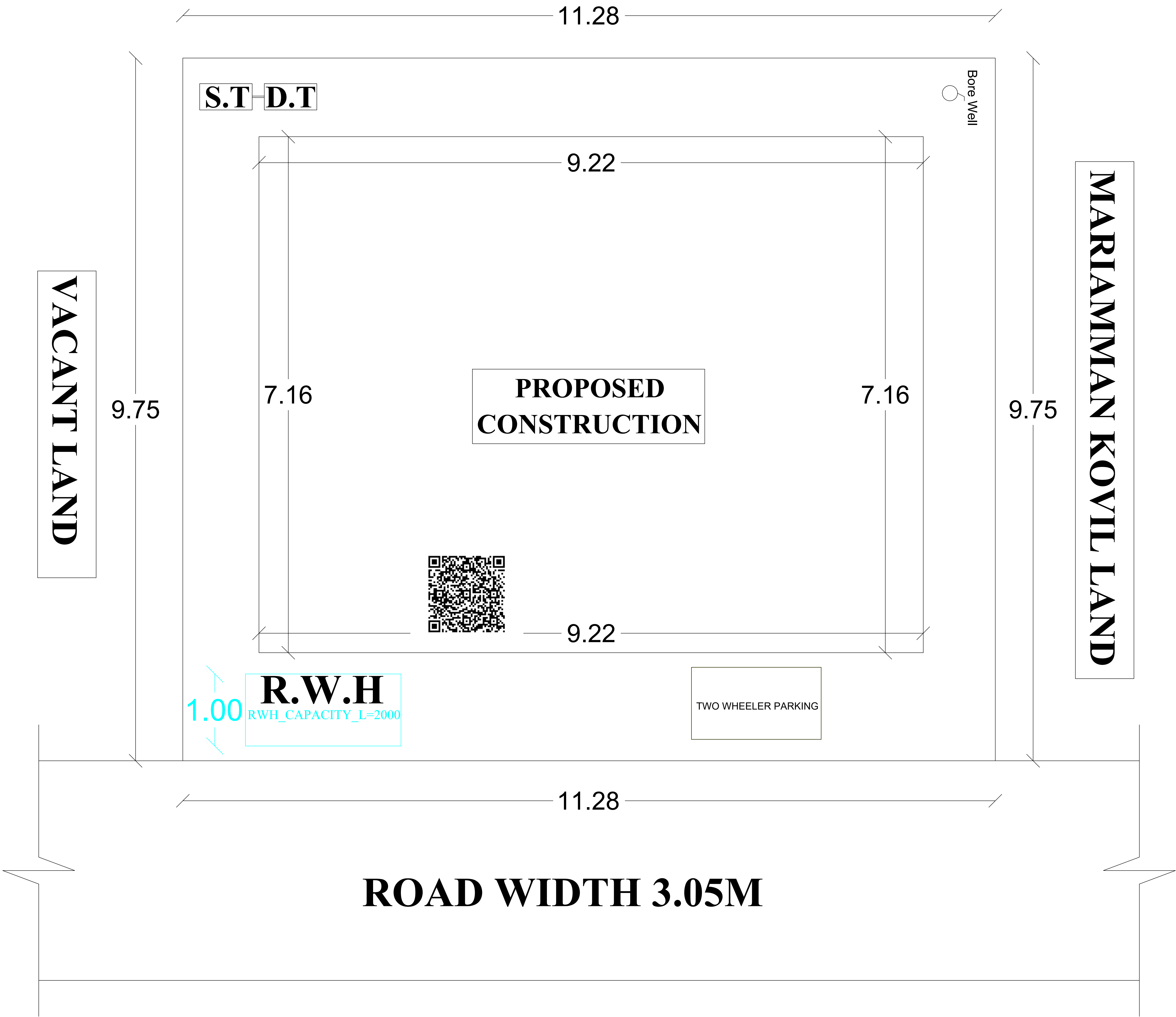
SITE PLAN ( Scale : 1:100 )
