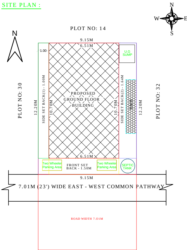
SITE PLAN :
