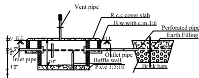
SECTION OF S.P.T & D.T
