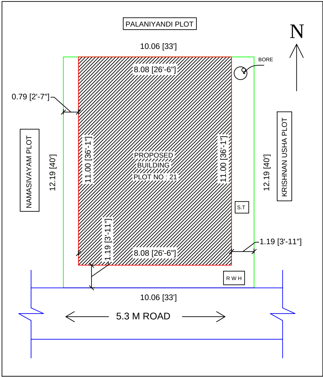
SITE PLAN 1:100
