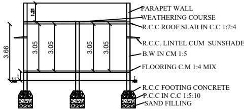
SECTION 'AB'
