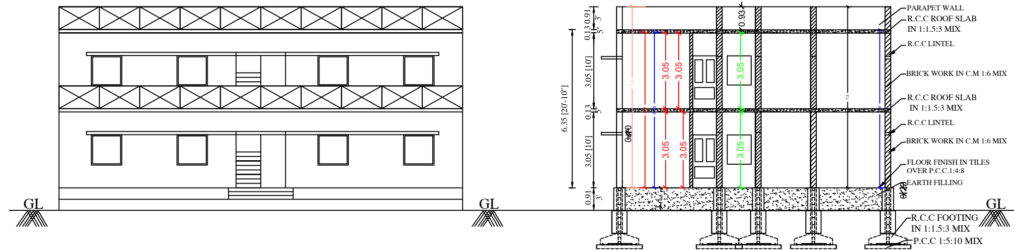
ELEVATION
