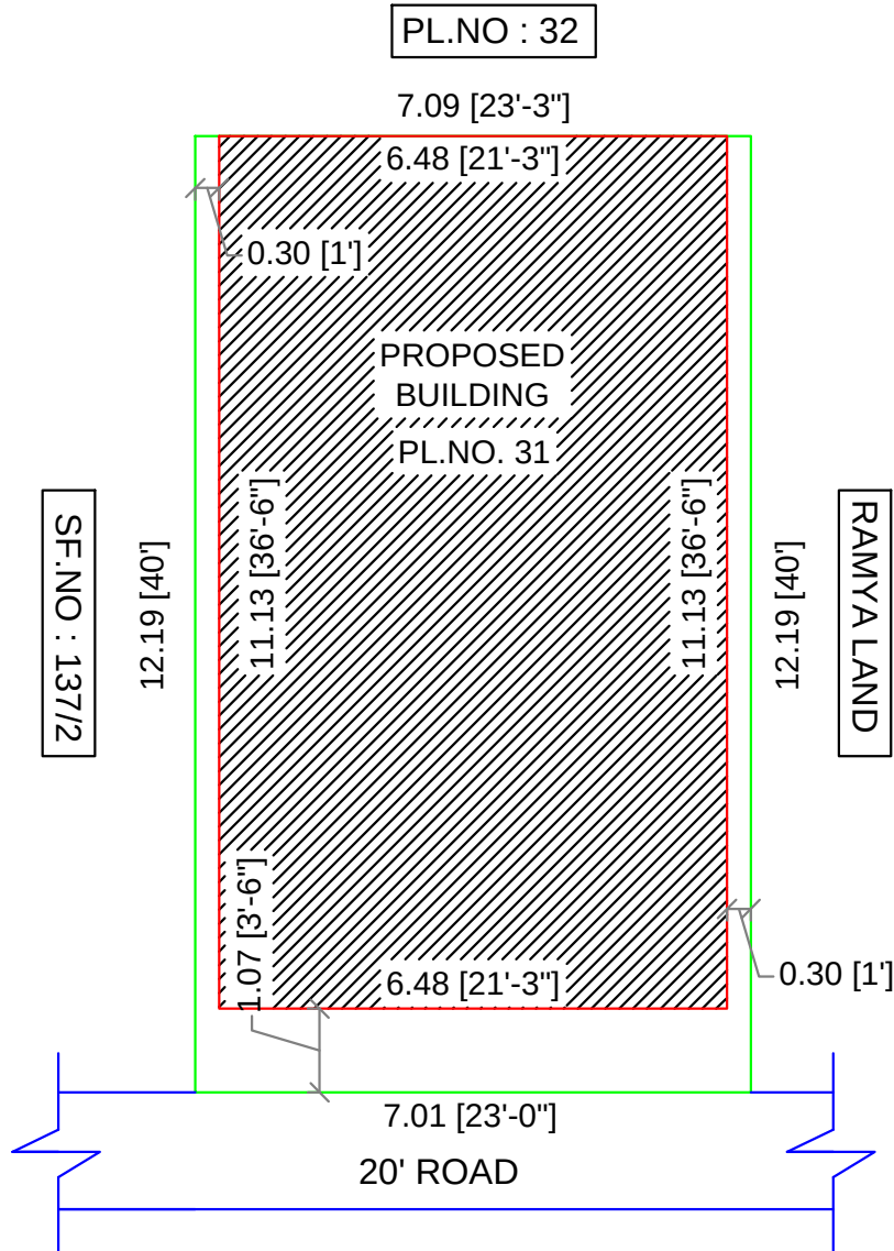
SITE PLAN 1:100
