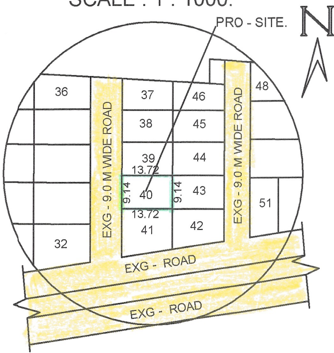
TOPO PLAN. SCALE : 1 : 1000.
