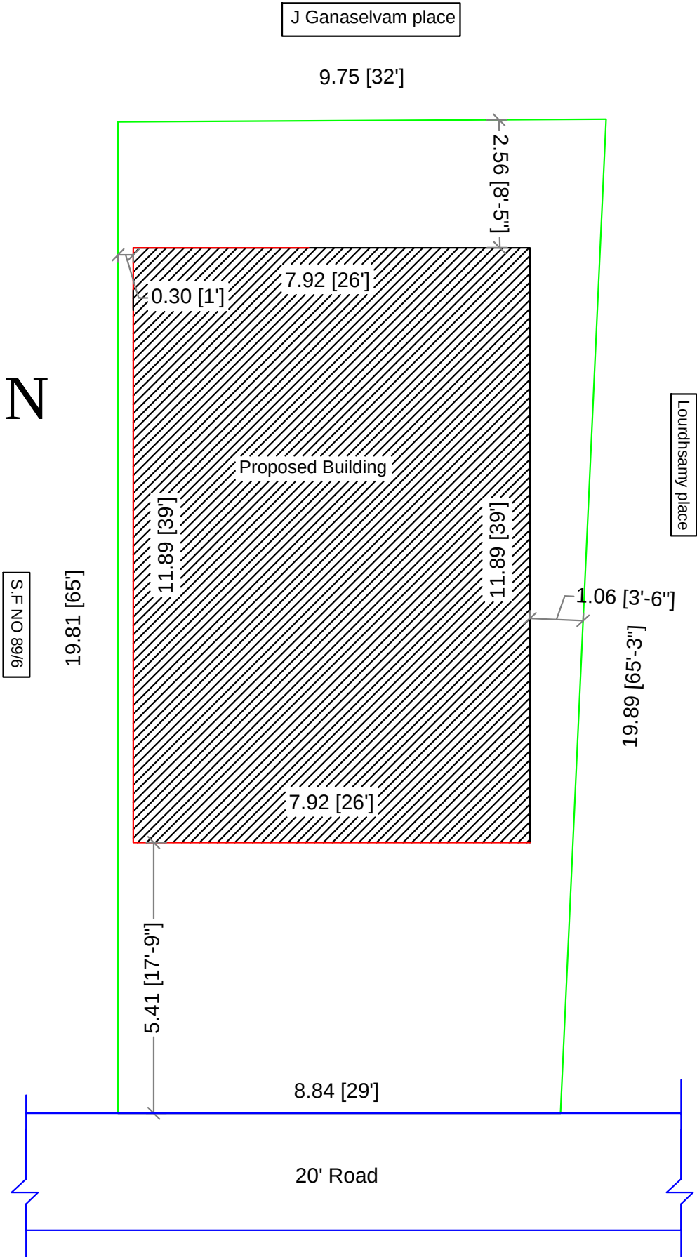
SITE PLAN 1:100
