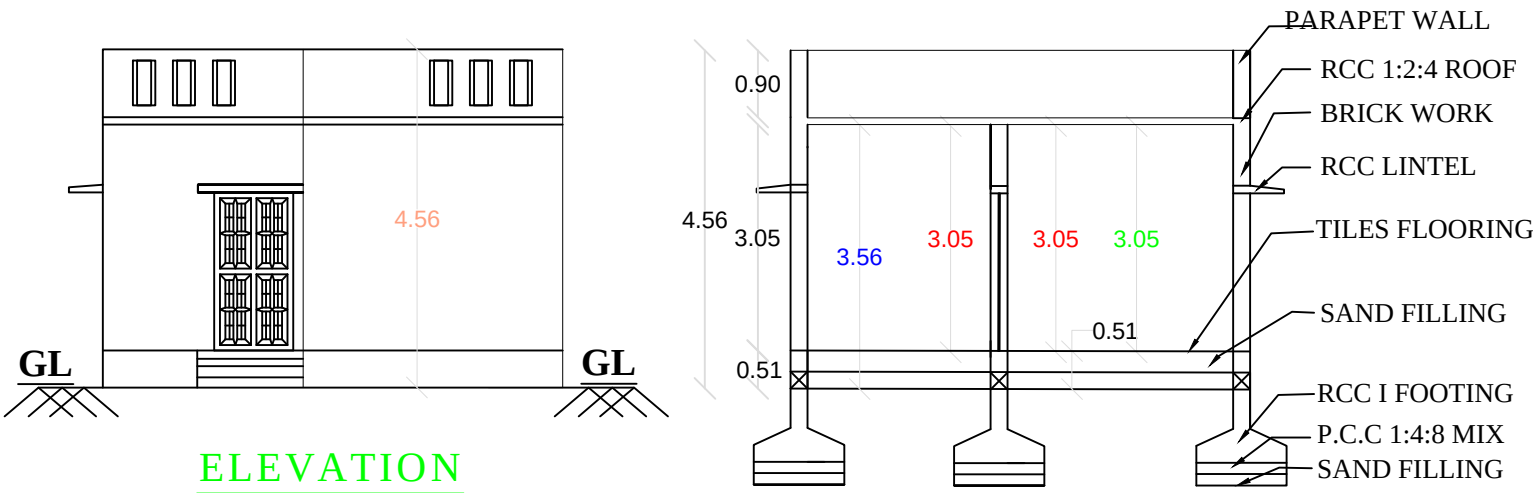
SECTION A-B
