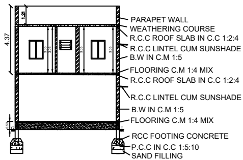
SECTION 'AB'
