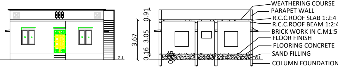
ELEVATION
