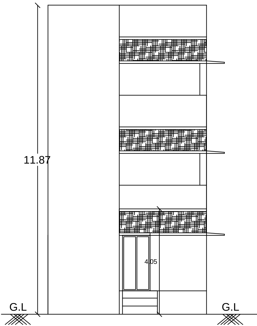
ELEVATION
