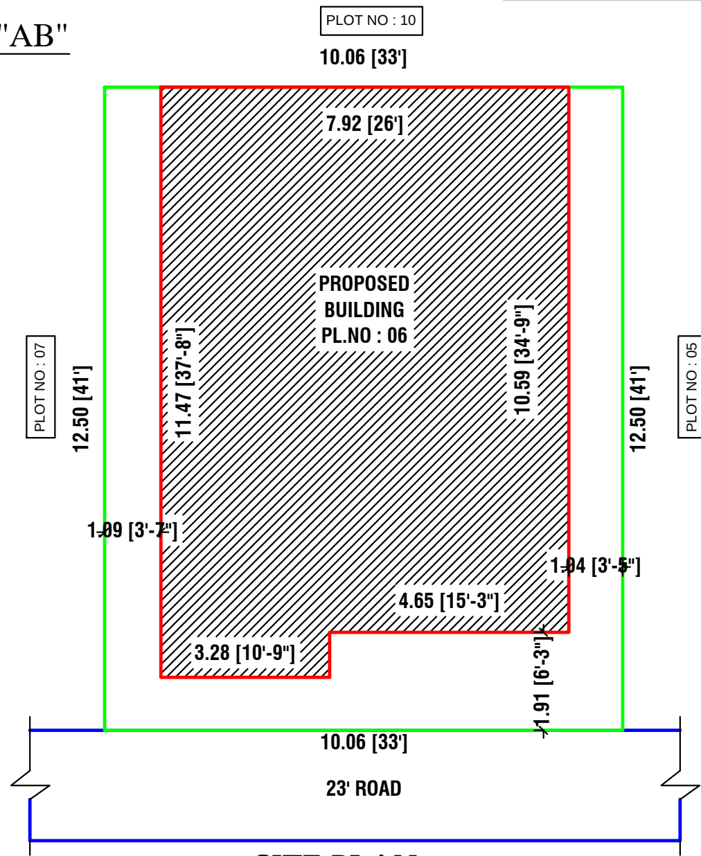
SITE PLAN 1:100
