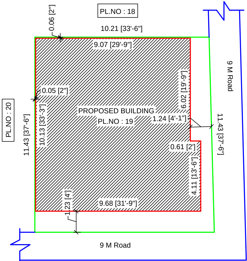
SITE PLAN ( 1: 100)
