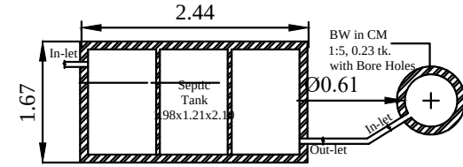
SOAK PIT
