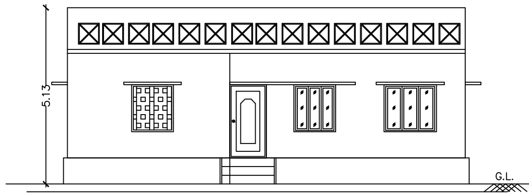
ELEVATION
