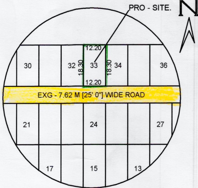
TOPO PLAN. SCALE : 1 : 1000.
