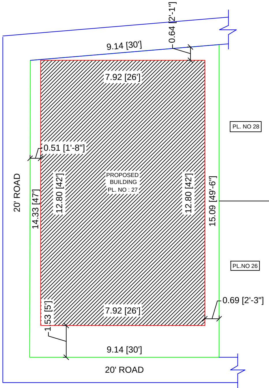
SITE PLAN ( 1:100)
