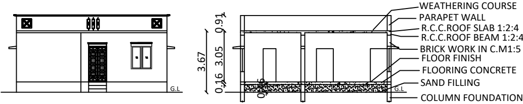
ELEVATION
