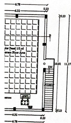
FLOOR PLAN SCALE: 1:100
