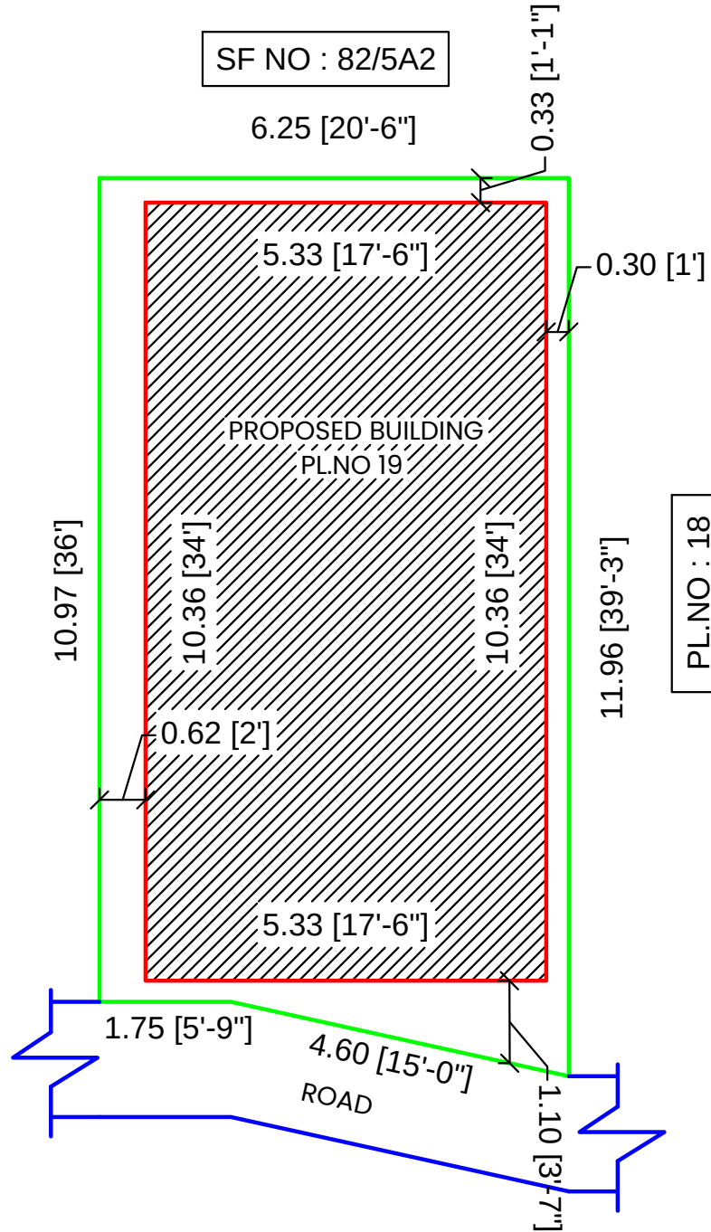
SITE PLAN ( 1:100)
