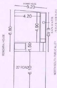
SITE PLAN SCALE 1:100
