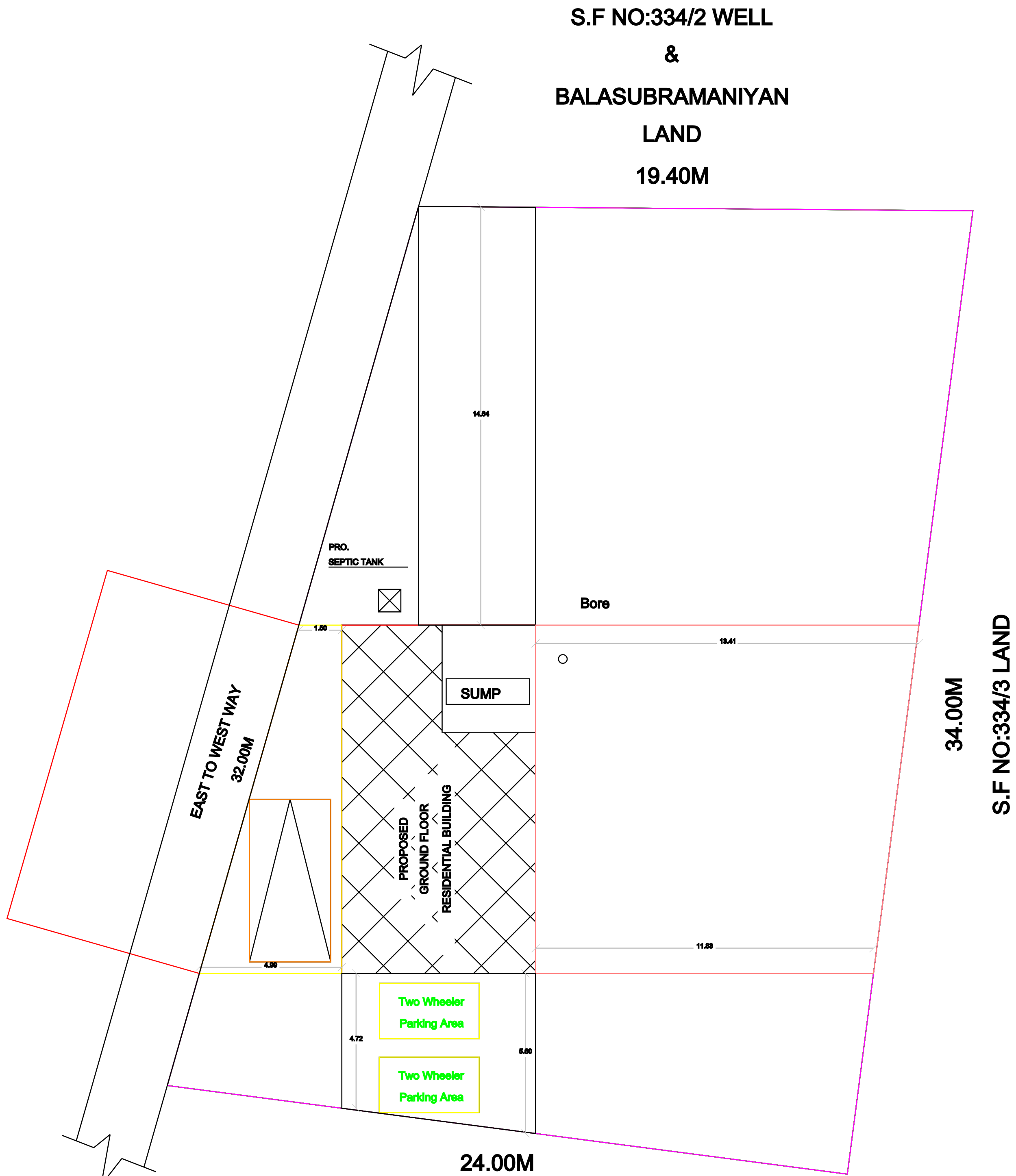
SITE PLAN (SCALE: 1:1)
