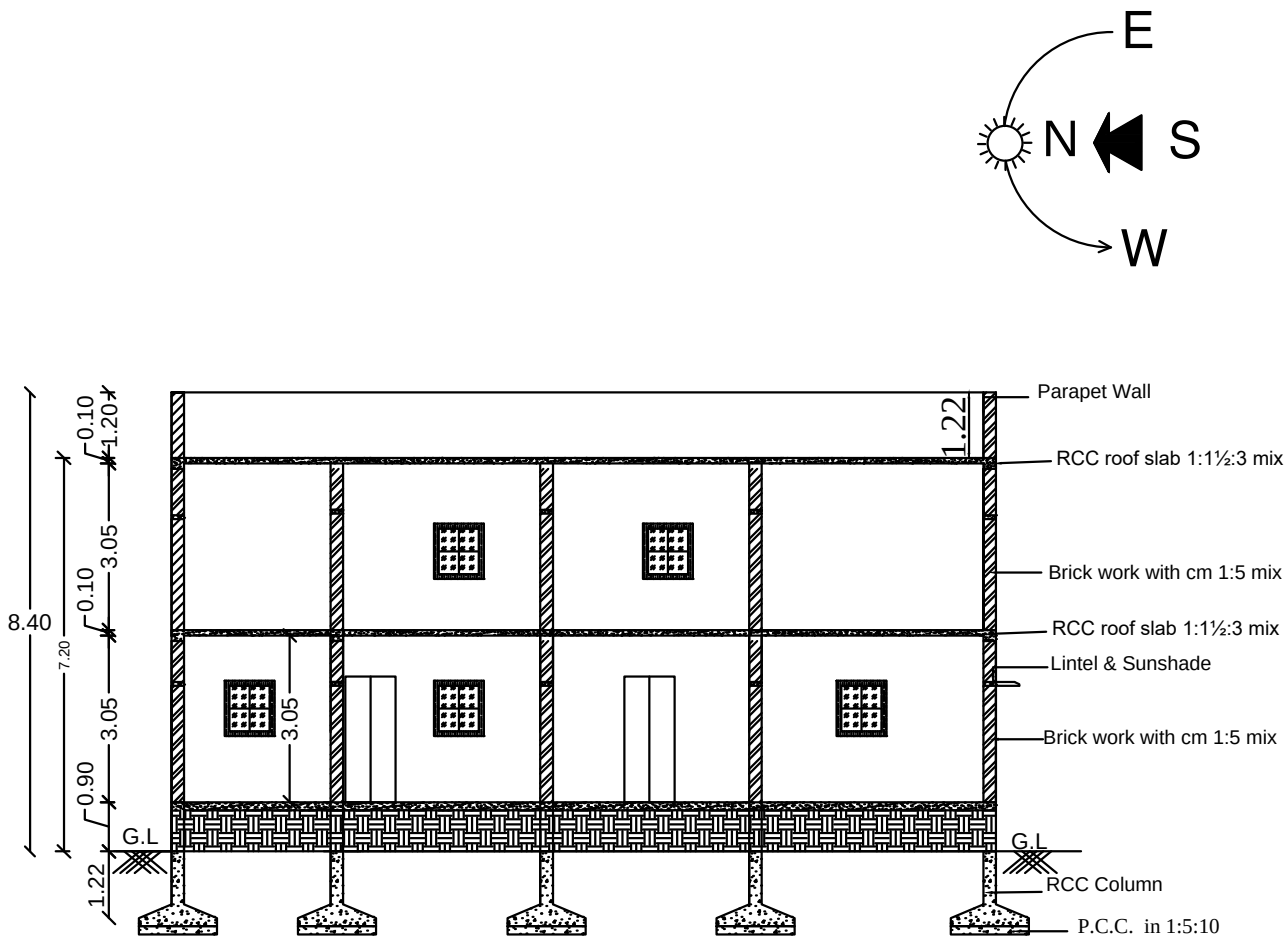
SECTION A-B
