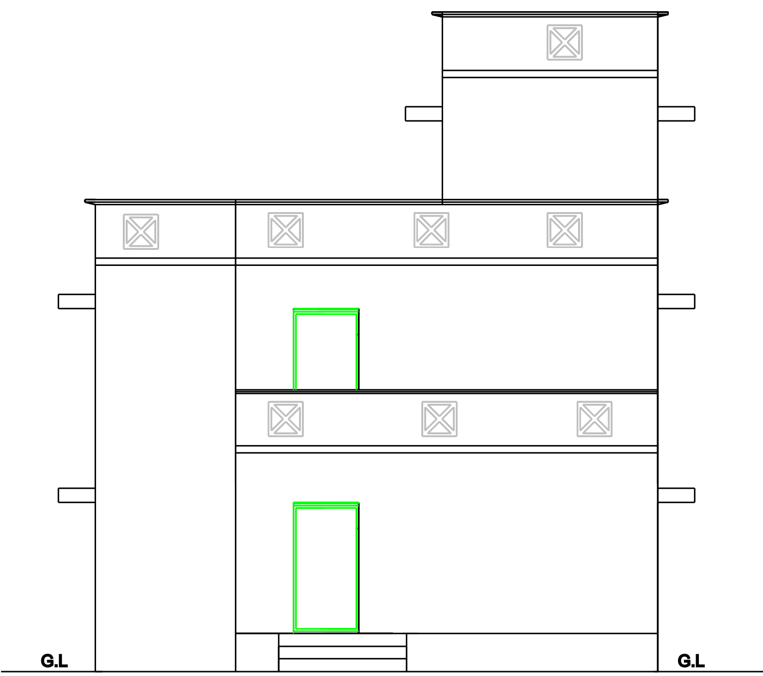
ELEVATION
