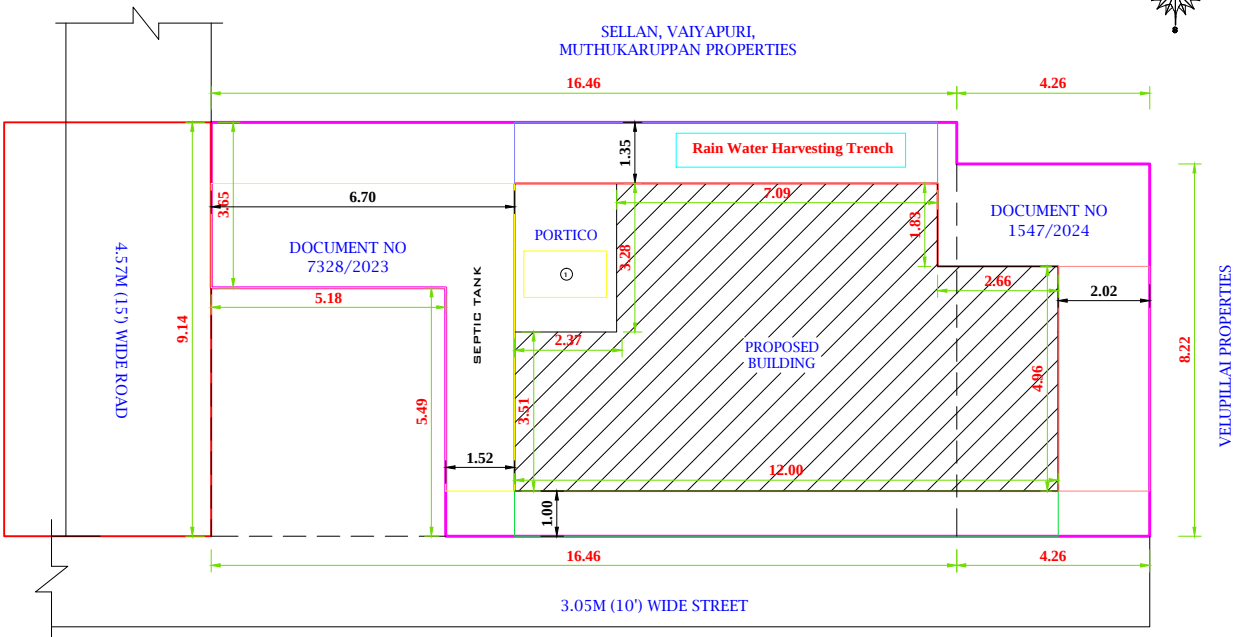
SITE PLAN 1:100
