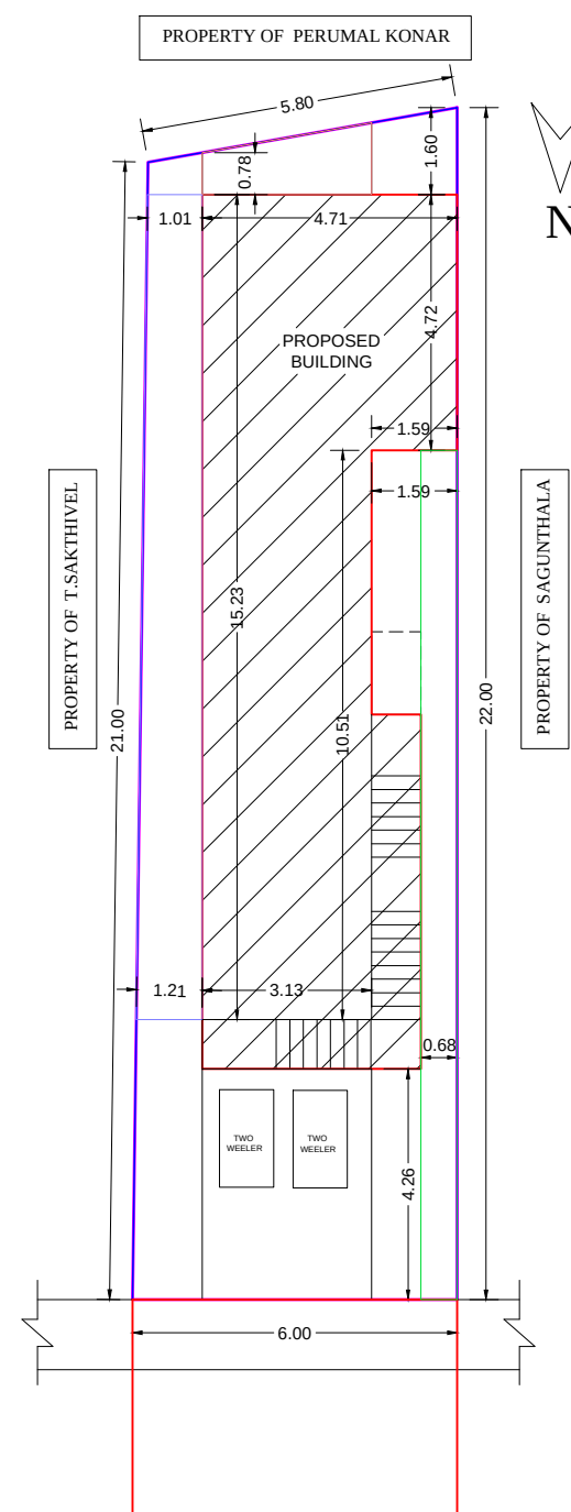
SITE PLAN 1:100
