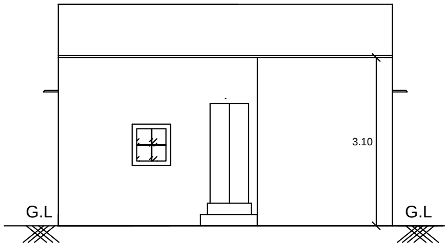
ELEVATION
