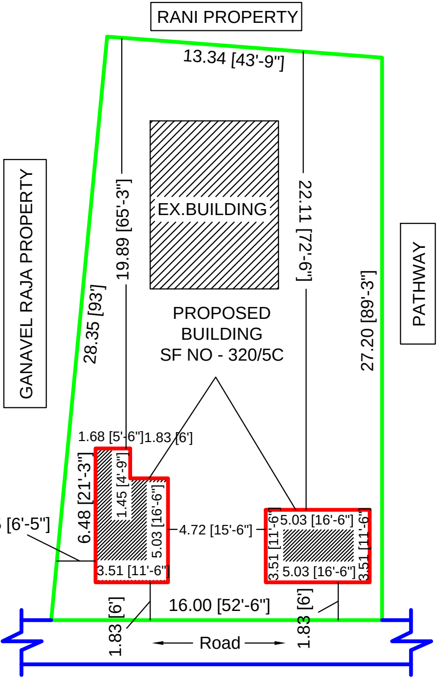
SITE PLAN (1:200)
