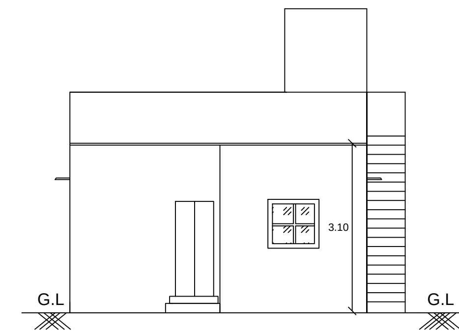
ELEVATION
