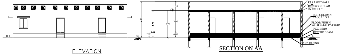
ELEVATION
