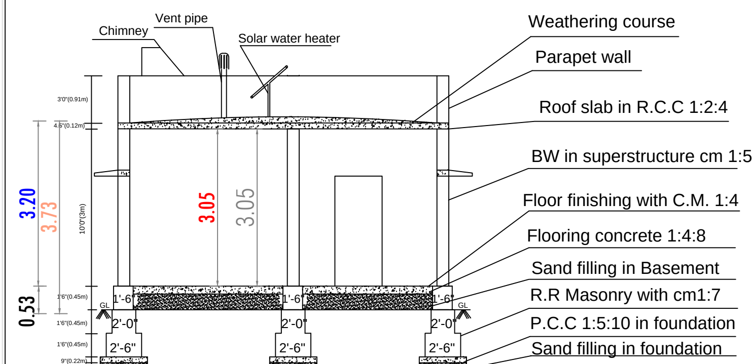
SECTION A-B
