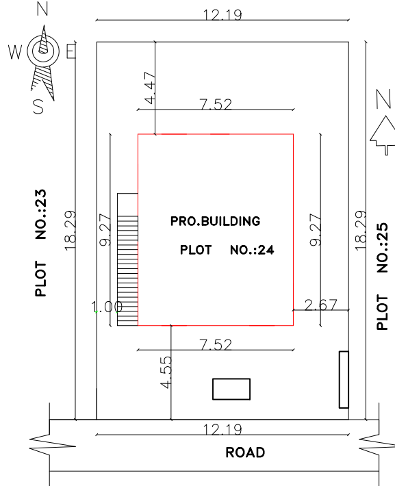
(SCALE 1: 100)
